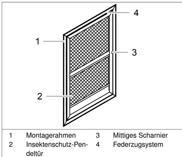
Abb. 1: Teileübersicht Insektenschutz-Pendeltür
