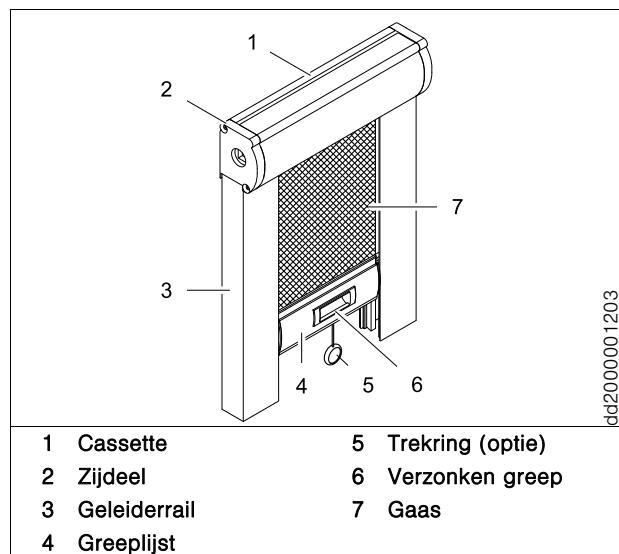
Afb. 1: Overzicht voor hor-rolgordijn
